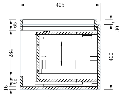
SEZIONE A-A
