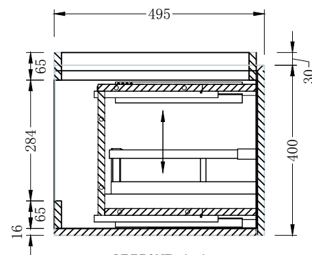
SEZIONE A-A
