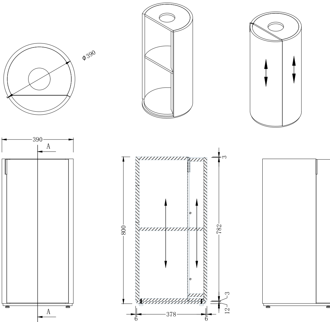
SEZIONE A-A
