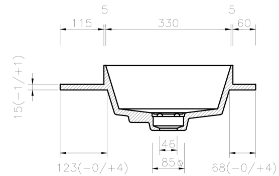
SEZIONE B-B SCALA 1:10
